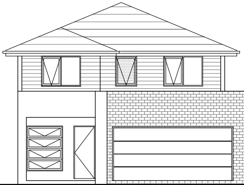
Elevation 1
