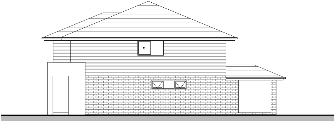
Elevation 3
